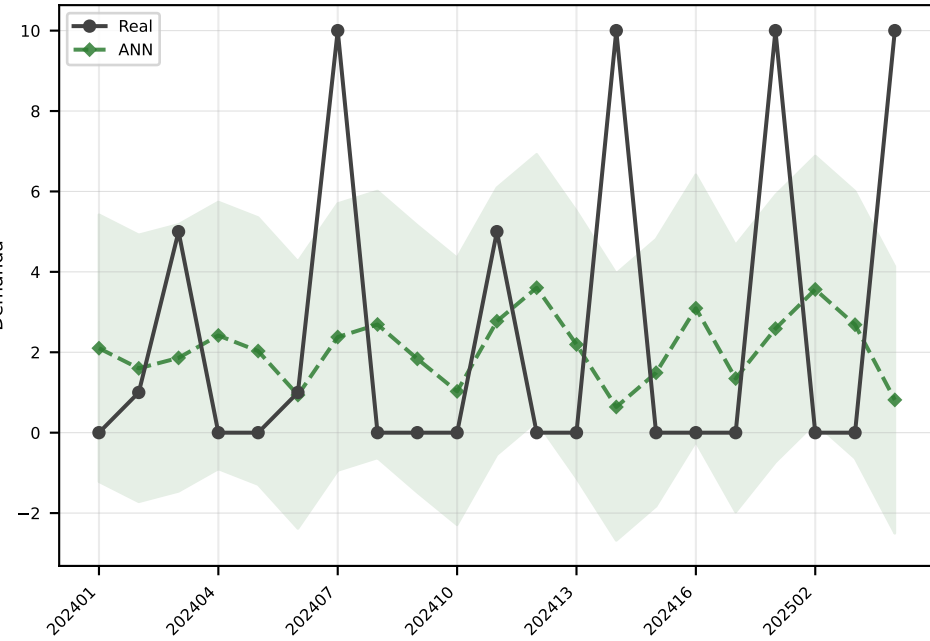
ANN MAE=3.3
