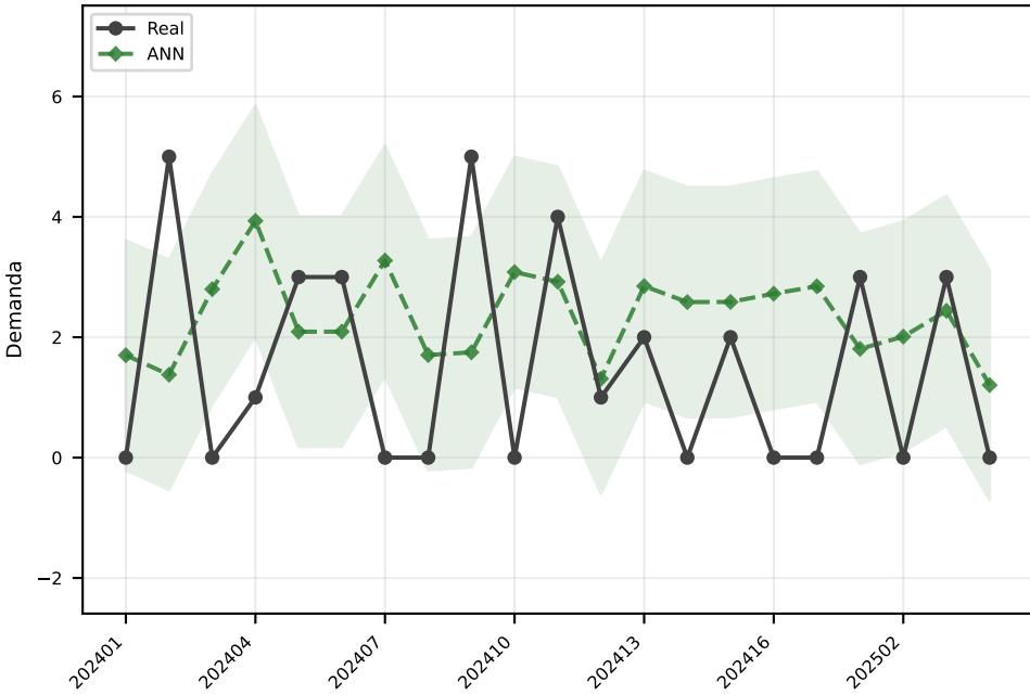
ANN MAE=1.9
