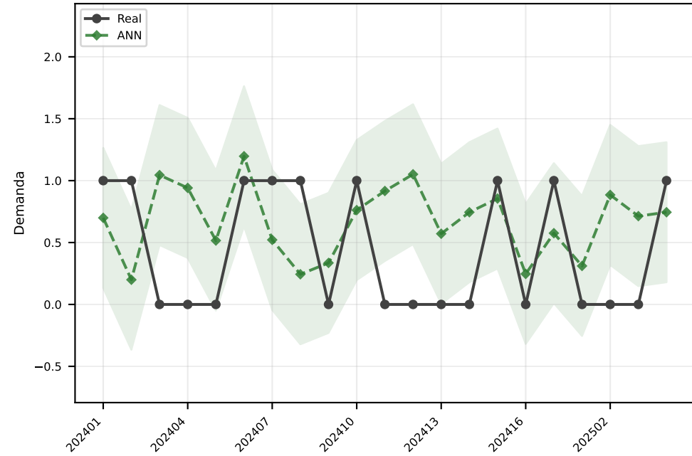
ANN MAE=0.6
