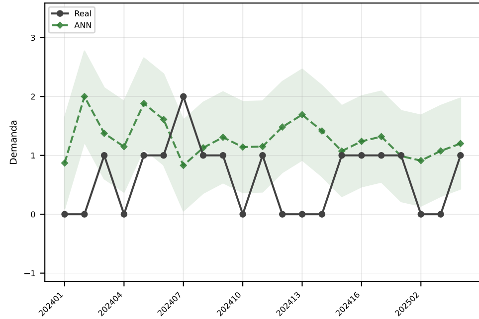
ANN MAE=0.8
