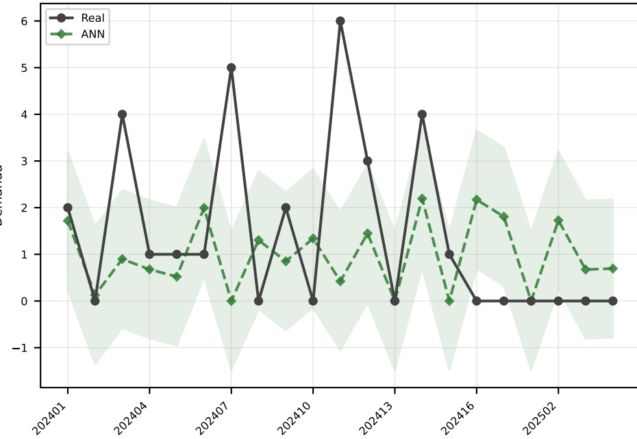
ANN MAE=1.5
