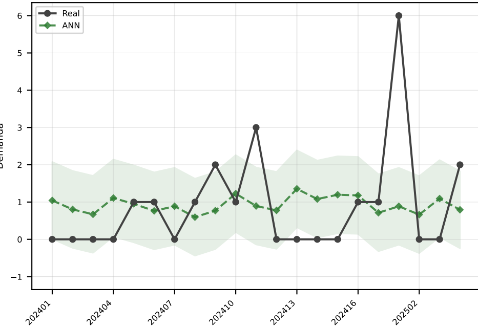
ANN MAE=1.0
