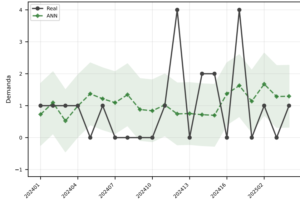
ANN MAE=1.0
