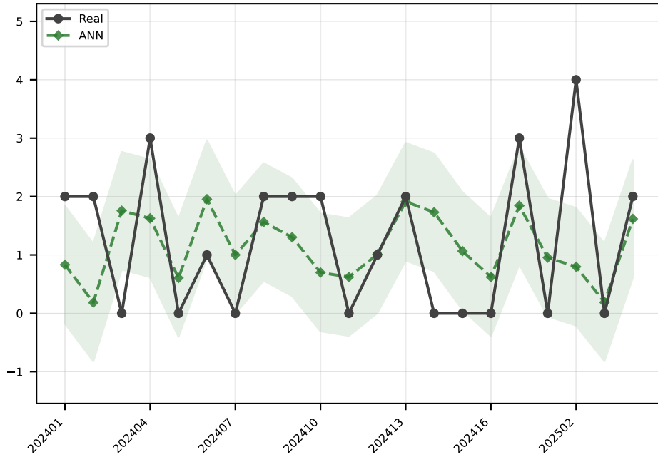
ANN MAE=1.0
