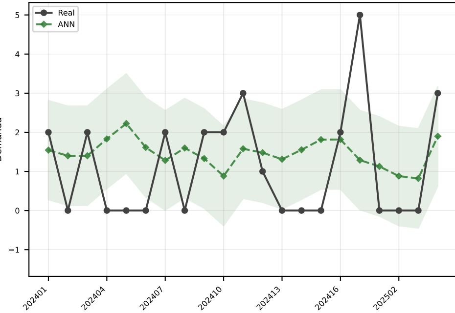
ANN MAE=1.3
