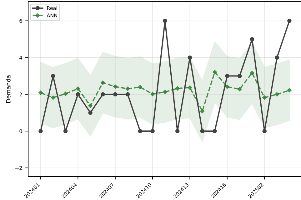
ANN MAE=1.6
