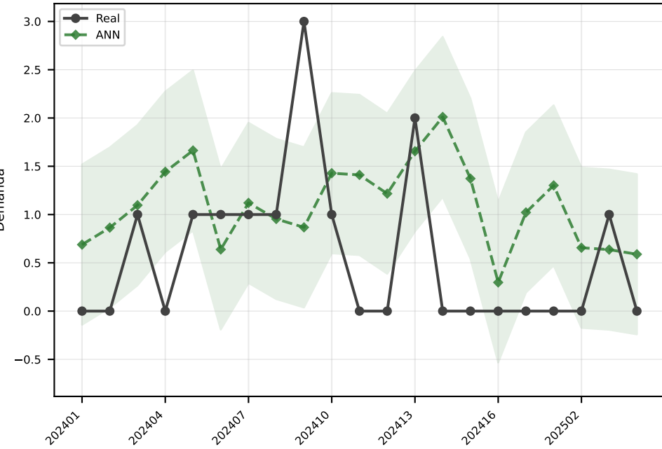
ANN MAE=0.8
