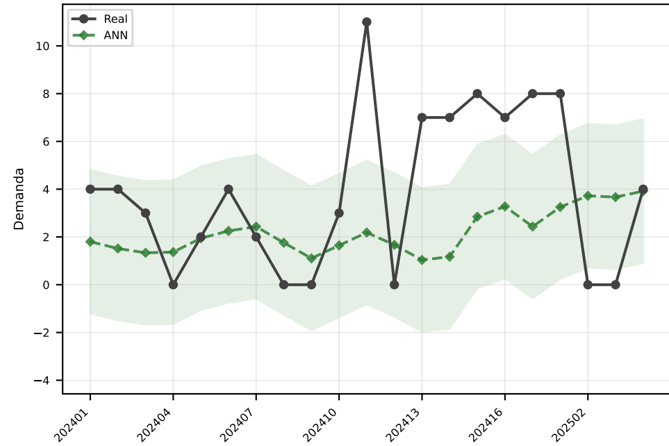
ANN MAE=3.0
