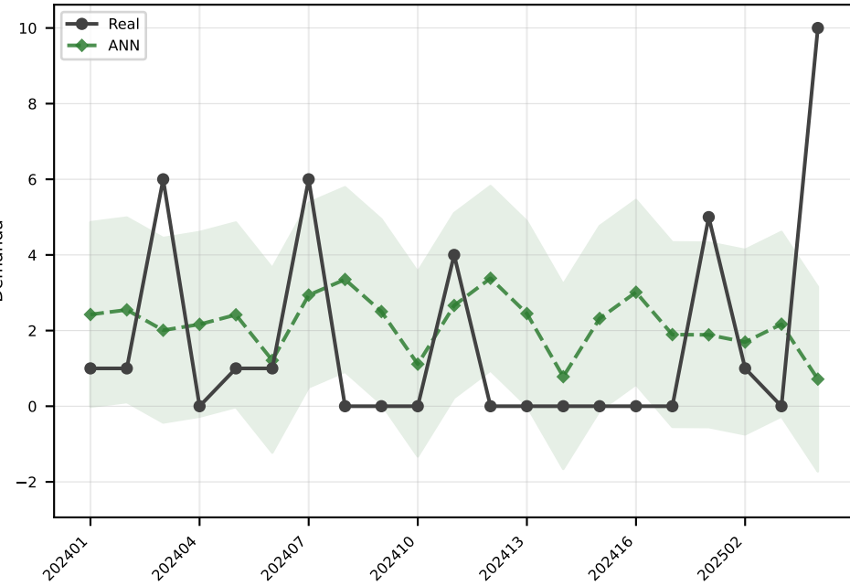
ANN MAE=2.4
