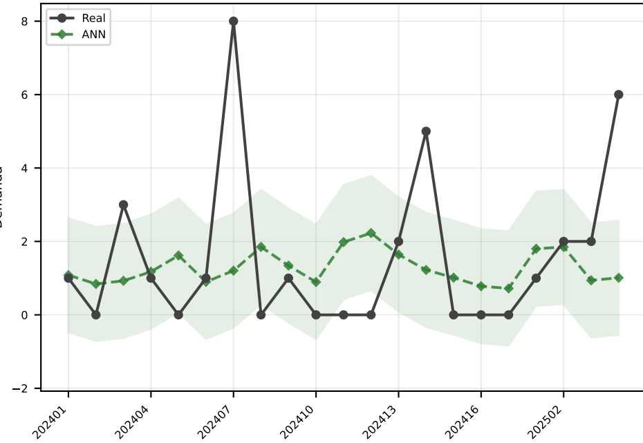
ANN MAE=1.6
