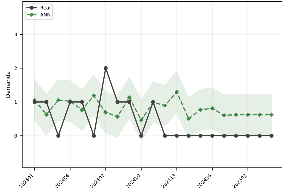
ANN MAE=0.6
