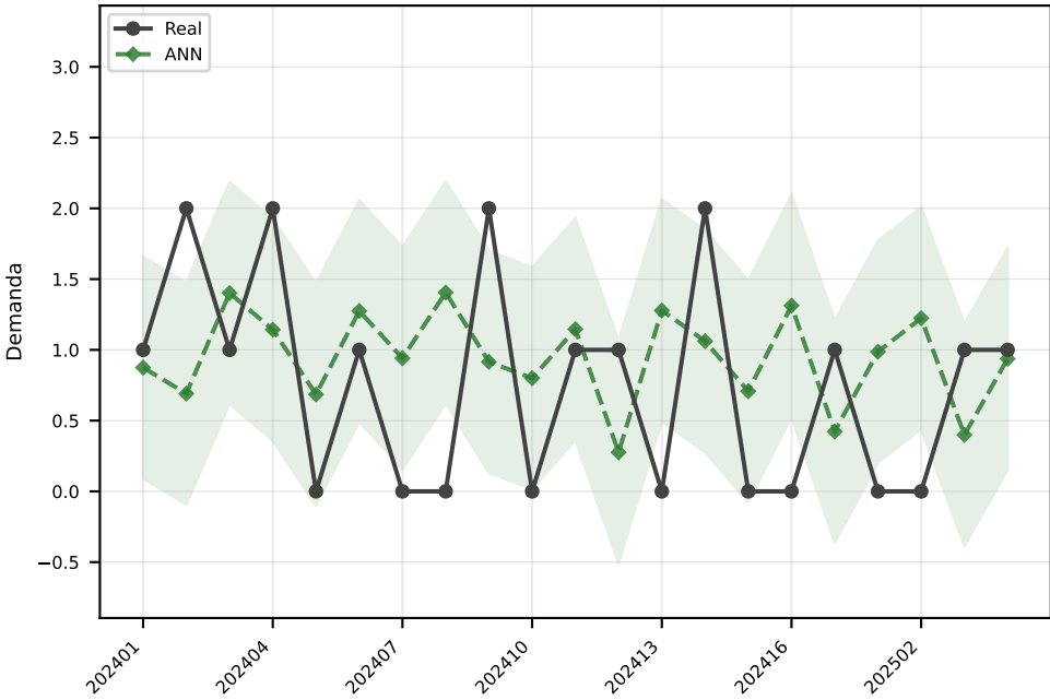
ANN MAE=0.8
