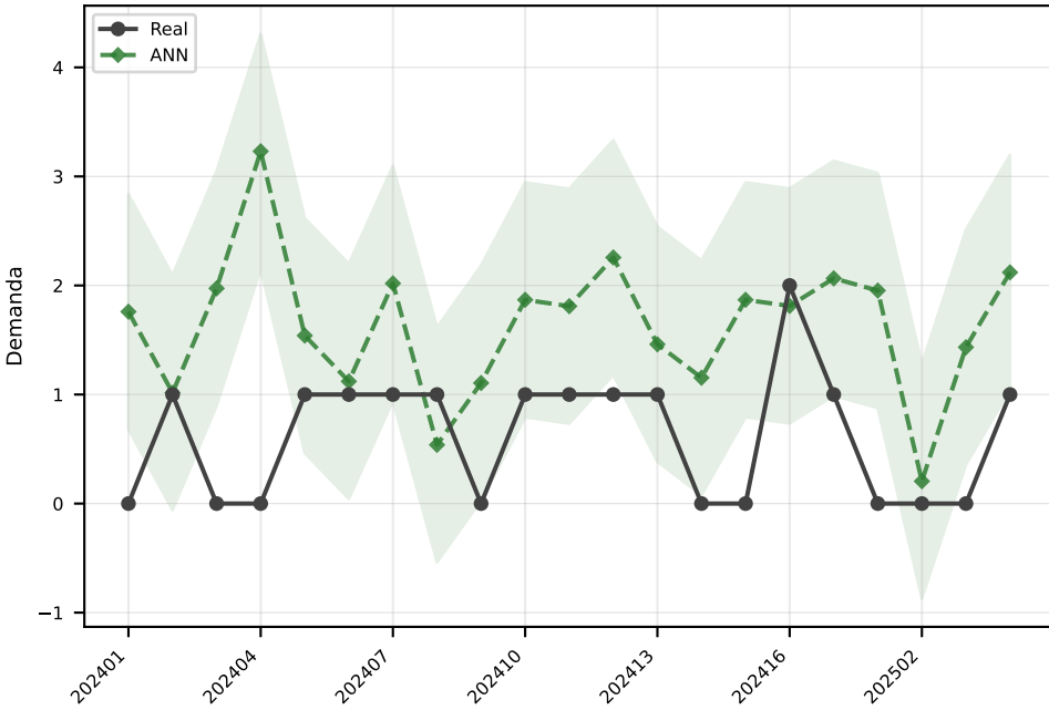
ANN MAE=1.1
