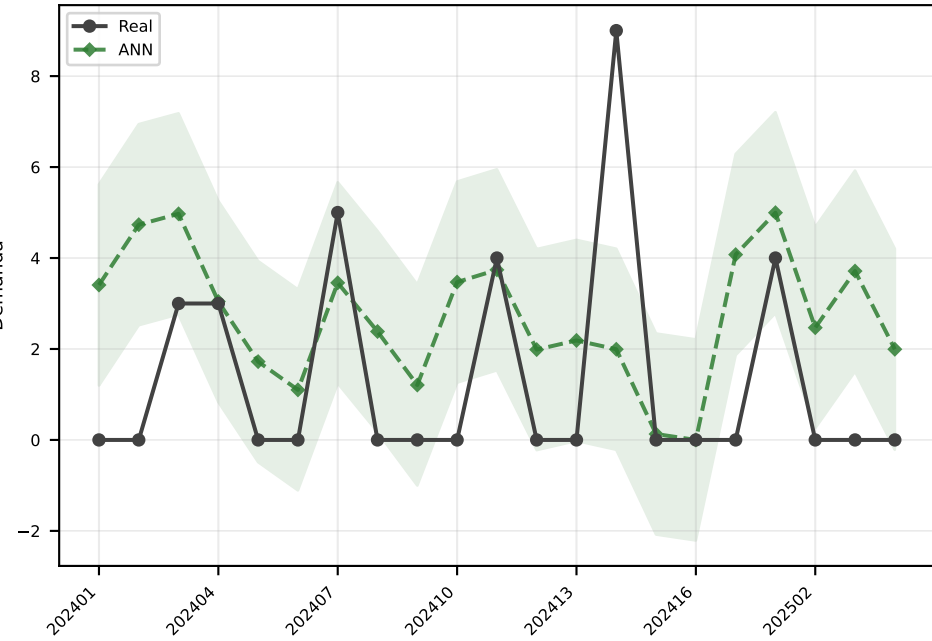
ANN MAE=2.2
