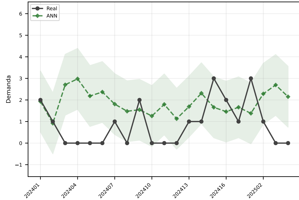
ANN MAE=1.4
