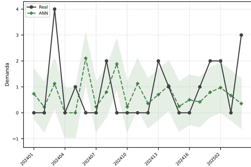
ANN MAE=1.0
