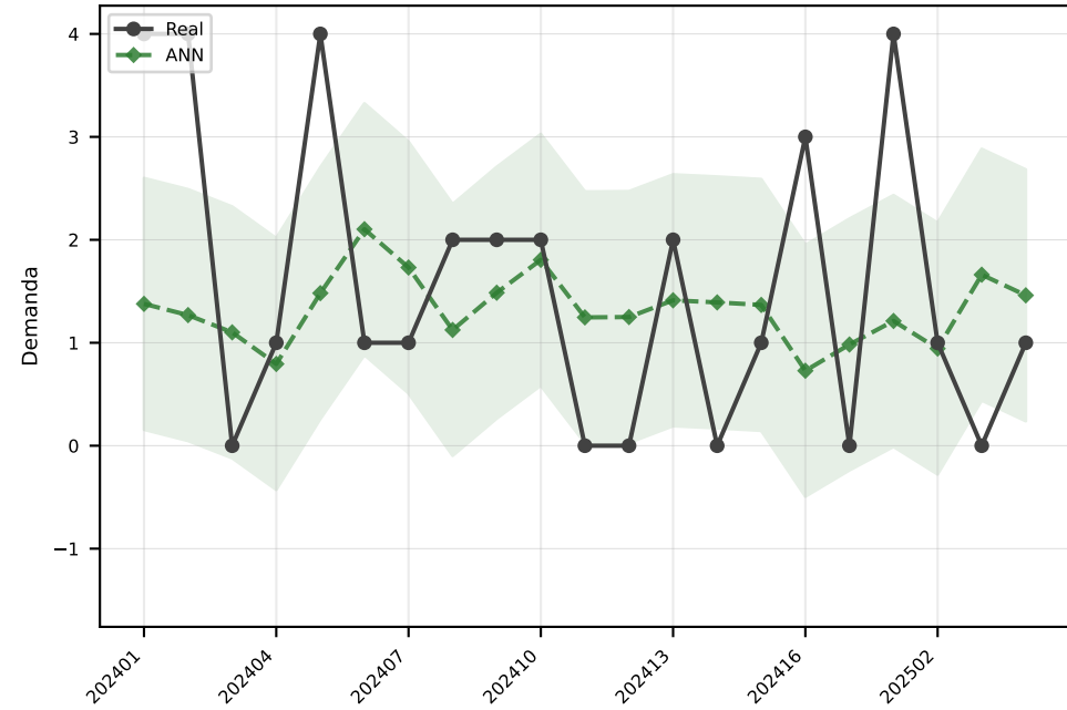
ANN MAE=1.2
