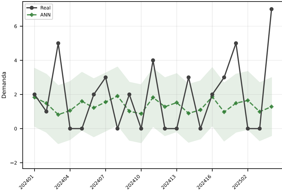
ANN MAE=1.7
