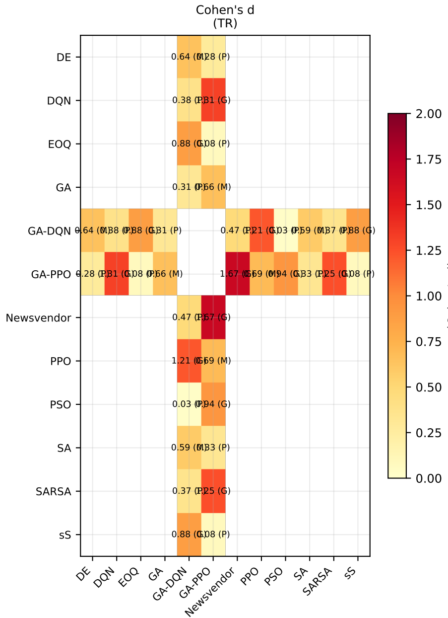
Tamanho de Efeito (Cohen's d) — G=grande, M=médio, P=pequeno
