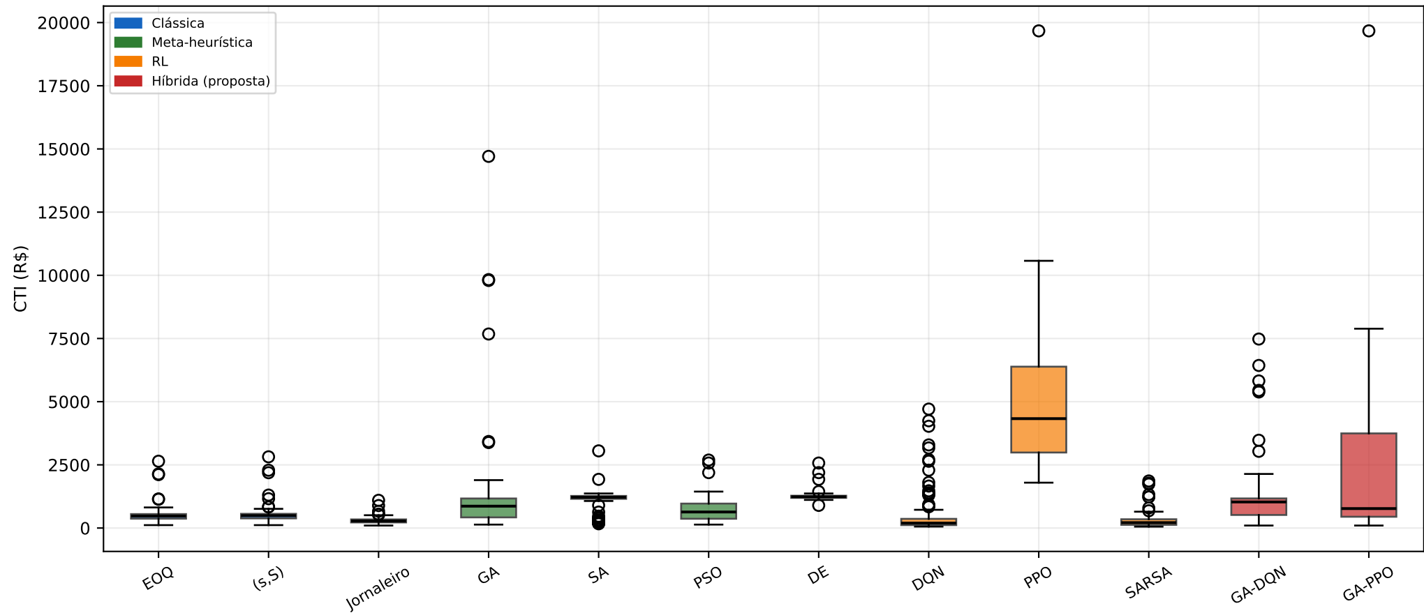
Distribuição do CTI por Política (todas as lojas × replicações)
