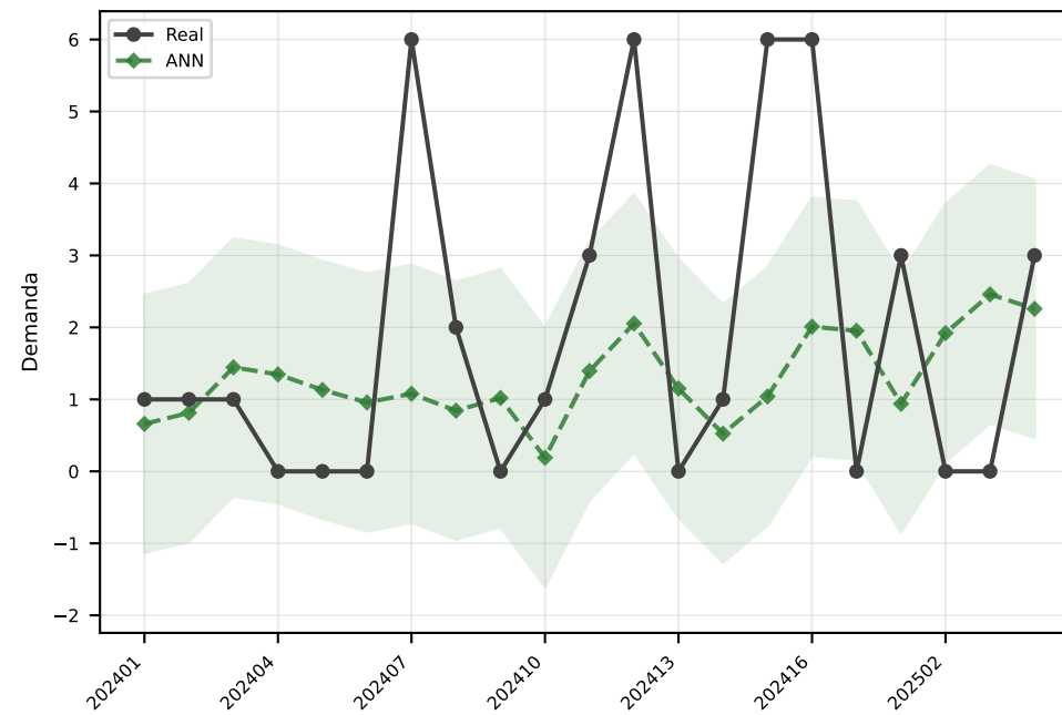
ANN MAE=1.8
