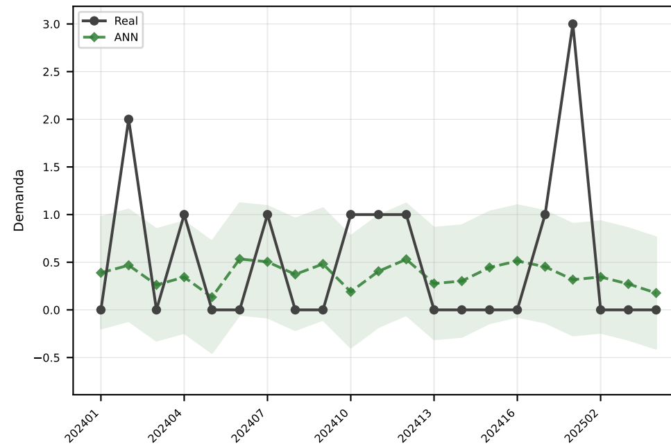
ANN MAE=0.6
