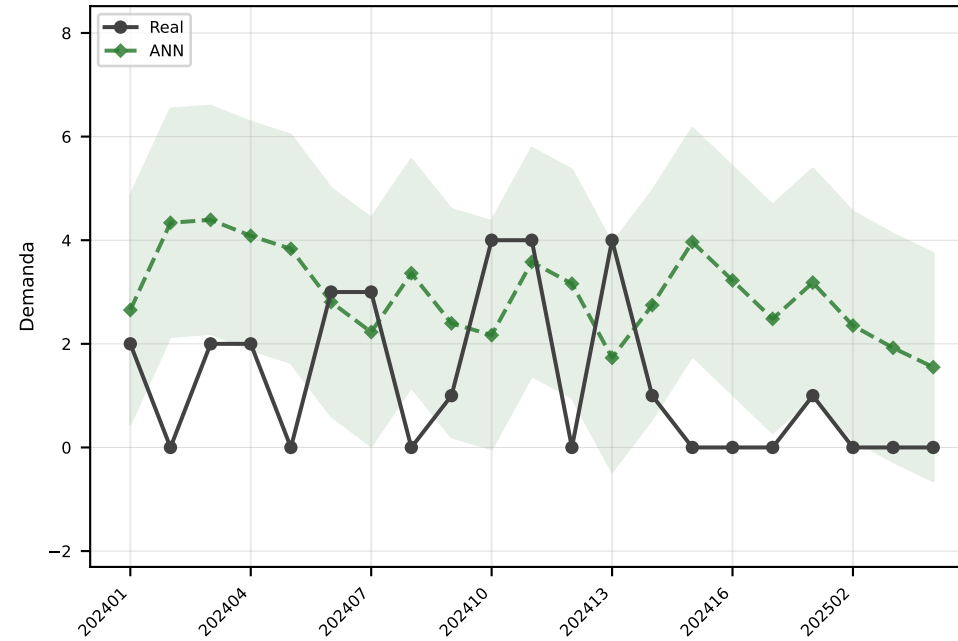
ANN MAE=2.2
