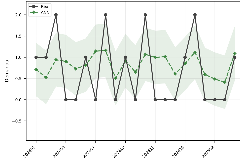
ANN MAE=0.6
