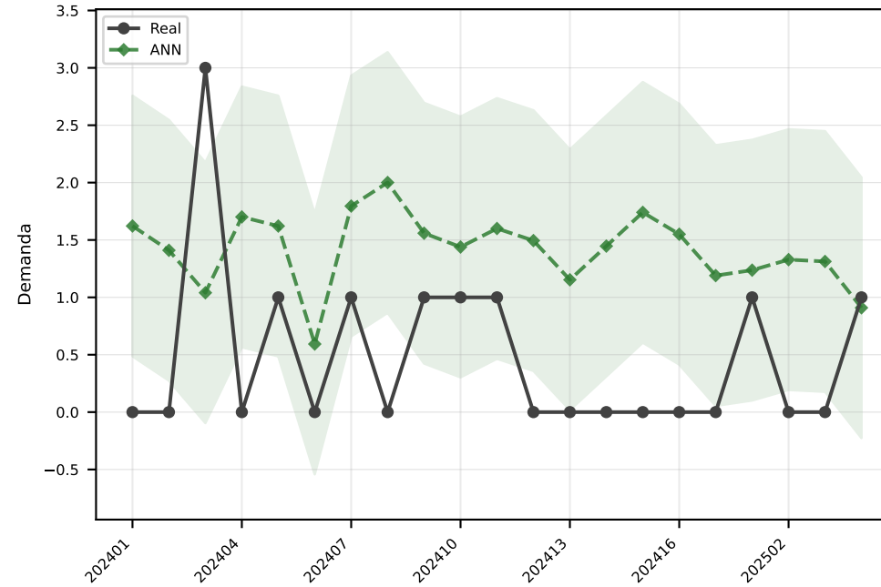
ANN MAE=1.1
