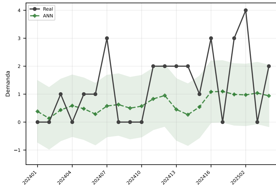
ANN MAE=1.1
