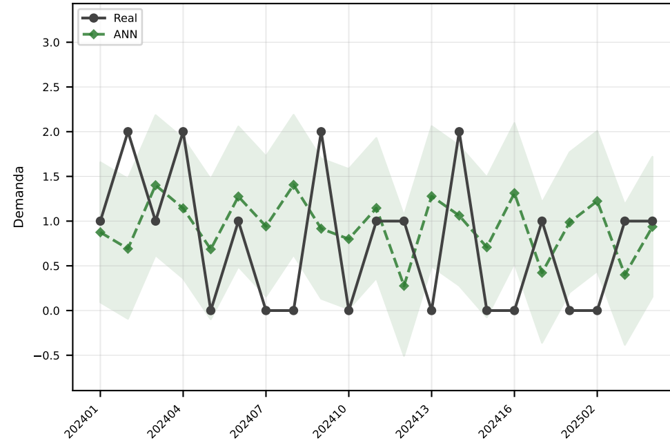
ANN MAE=0.8
