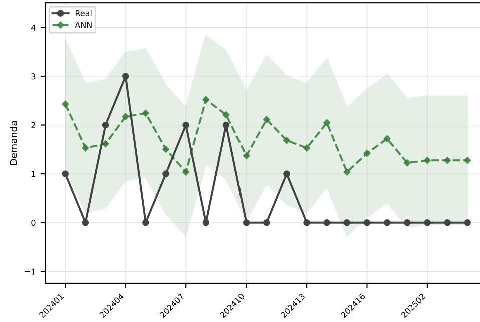
ANN MAE=1.3
