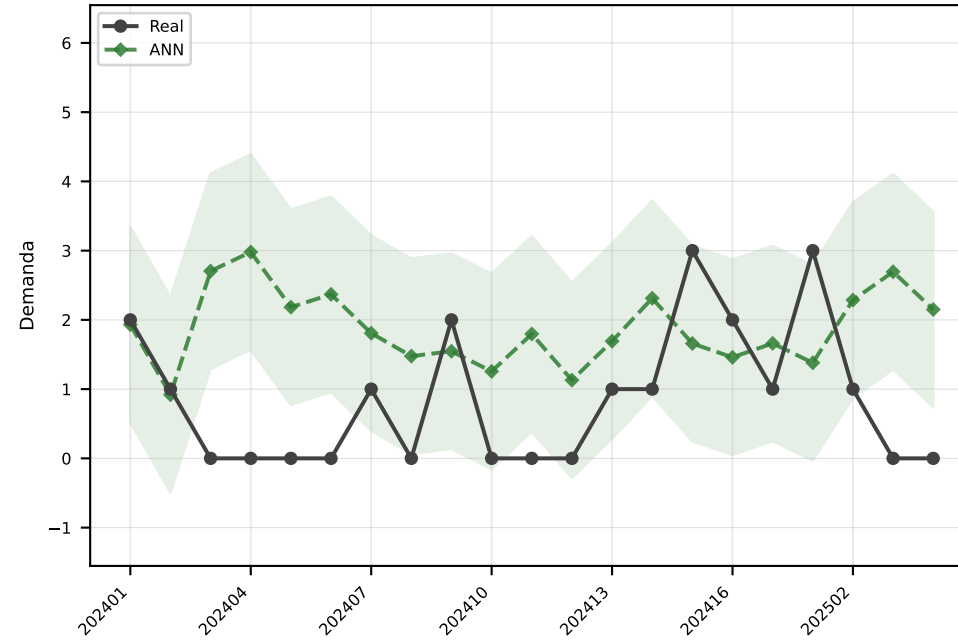
ANN MAE=1.4
