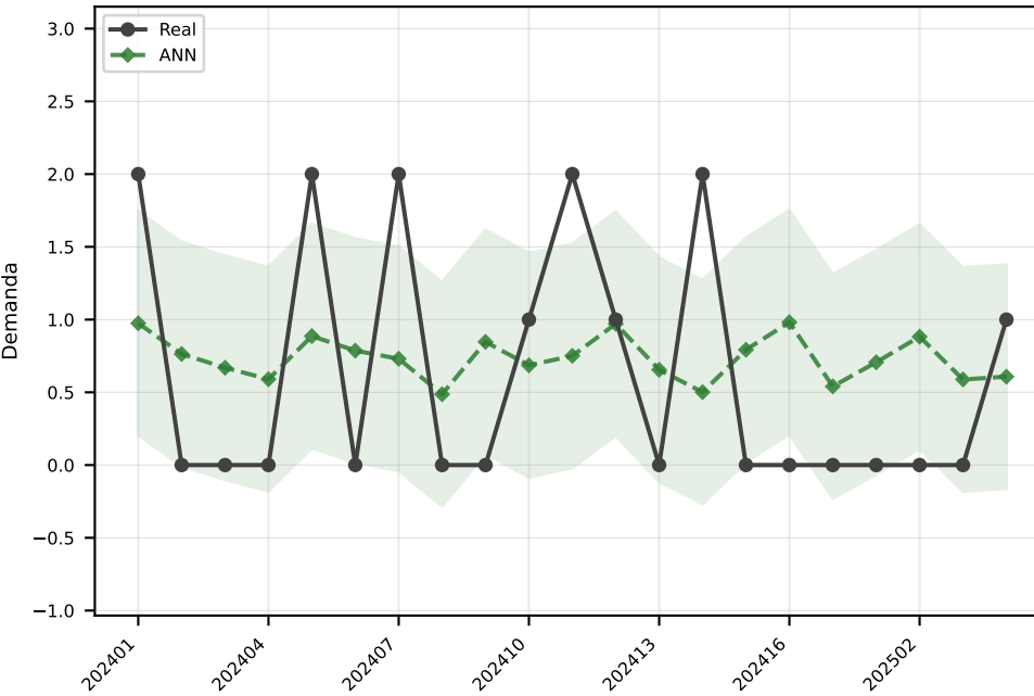
ANN MAE=0.8
