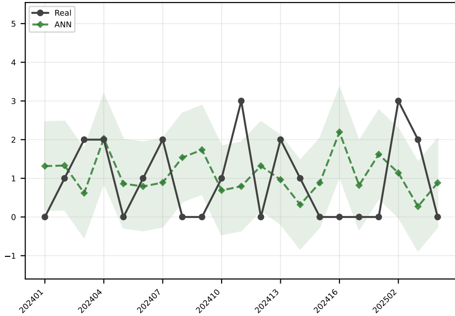
ANN MAE=1.1
