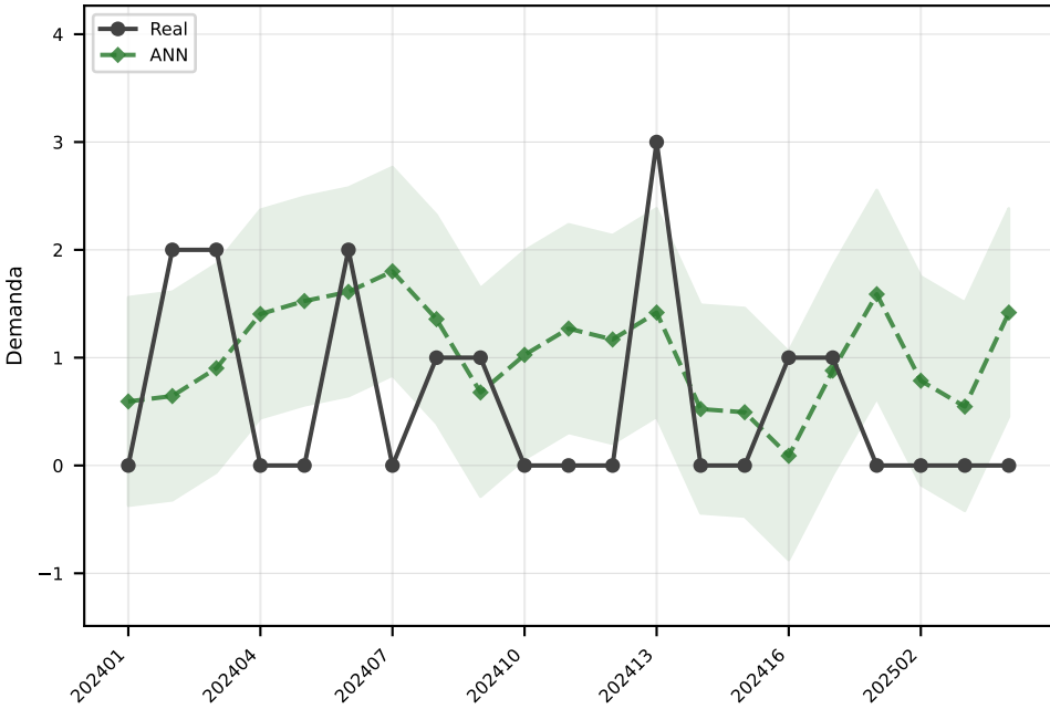
ANN MAE=1.0
