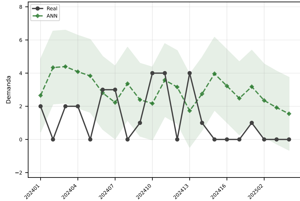
ANN MAE=2.2
