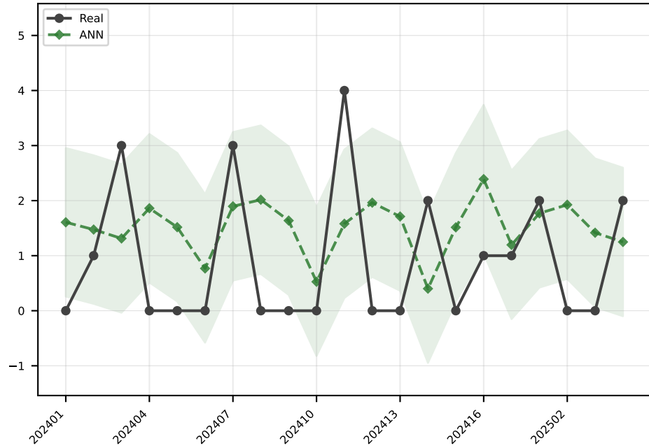
ANN MAE=1.3
