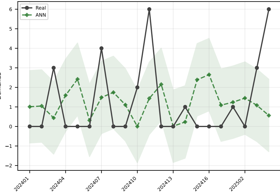
ANN MAE=1.9
