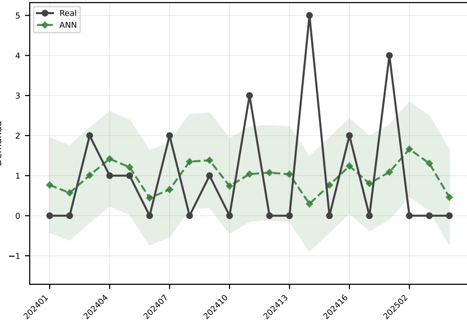
ANN MAE=1.2
