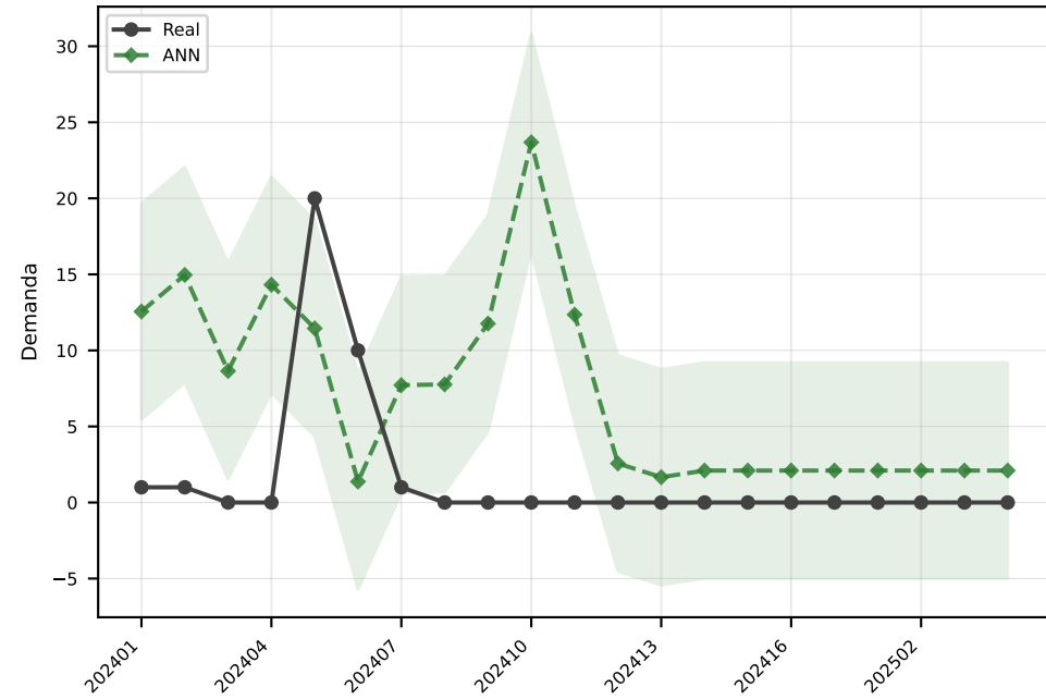
ANN MAE=7.1
