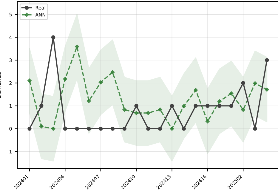
ANN MAE=1.4
