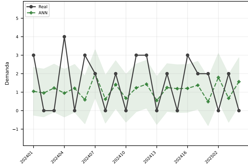
ANN MAE=1.3
