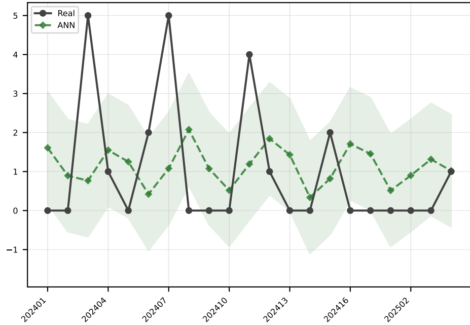
ANN MAE=1.4
