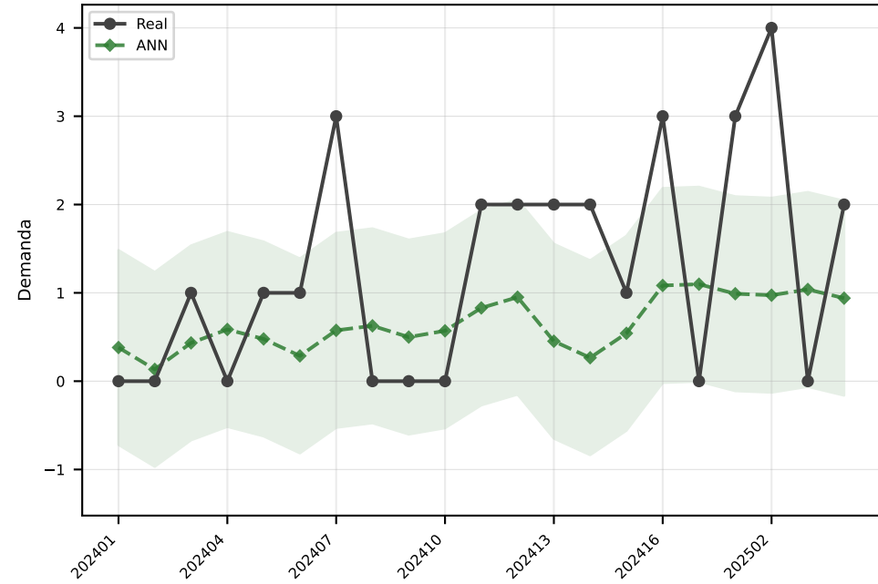
ANN MAE=1.1
