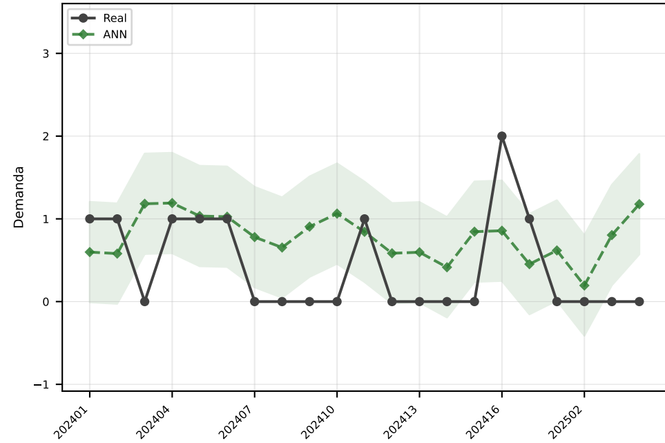
ANN MAE=0.6
