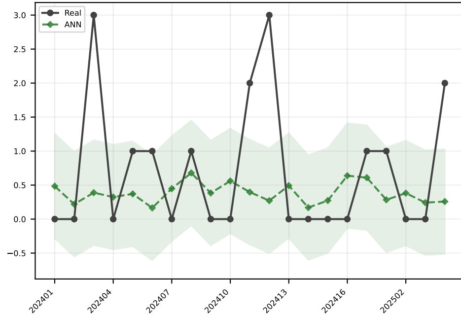
ANN MAE=0.8
