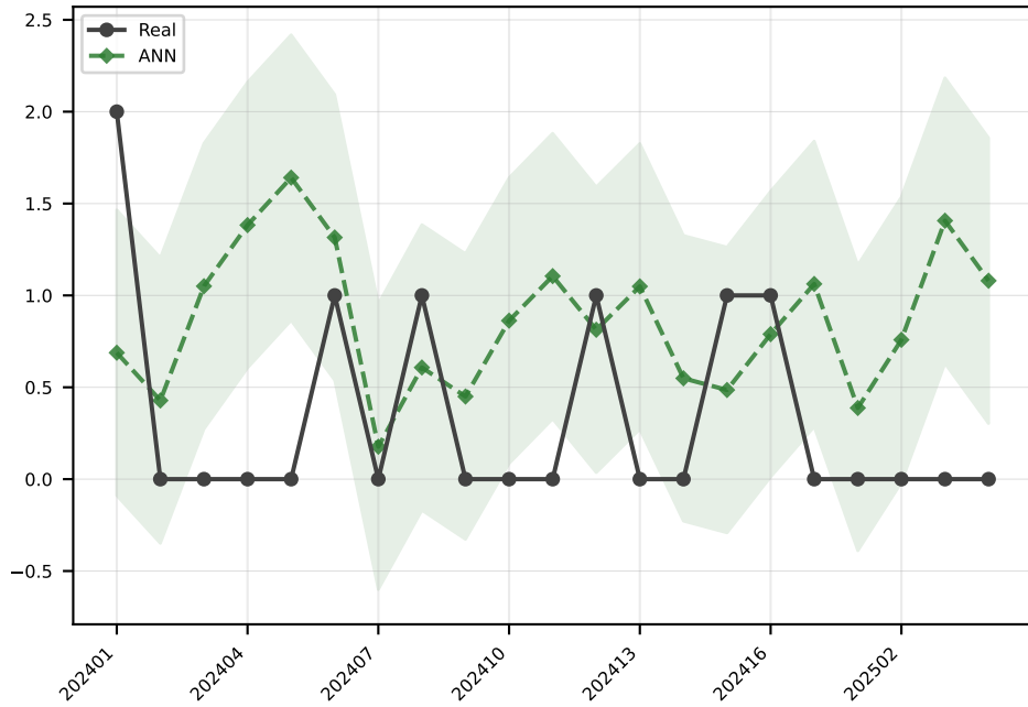
ANN MAE=0.8
