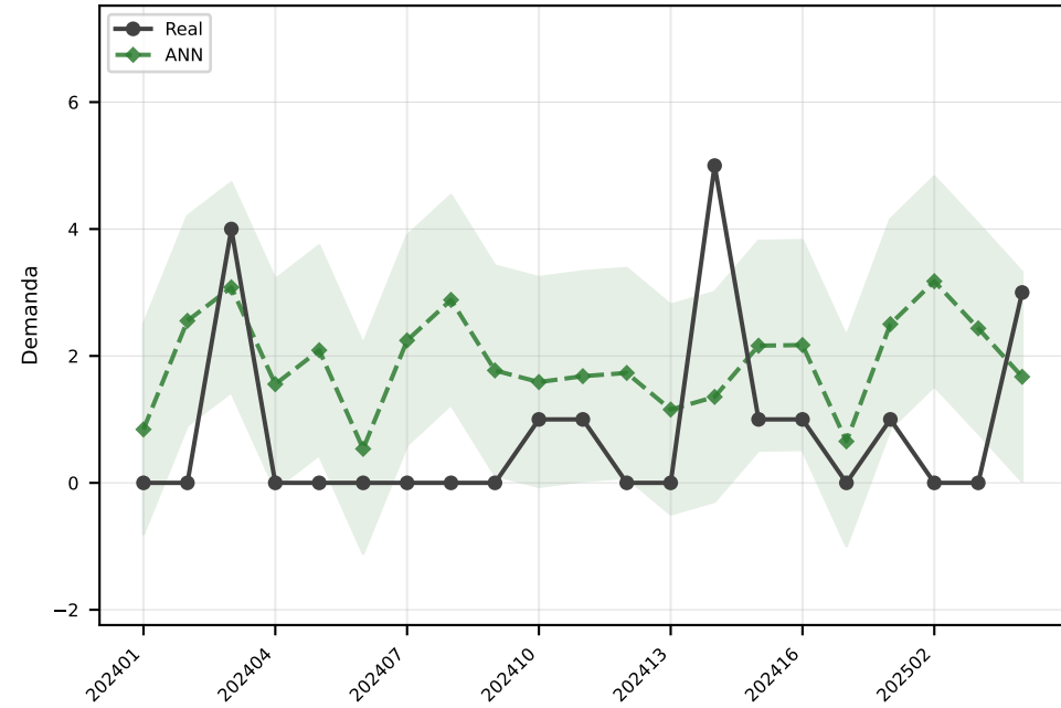
ANN MAE=1.6
