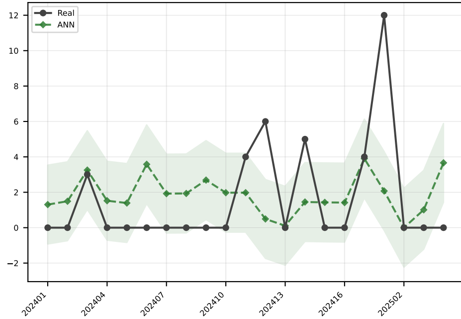
ANN MAE=2.2
